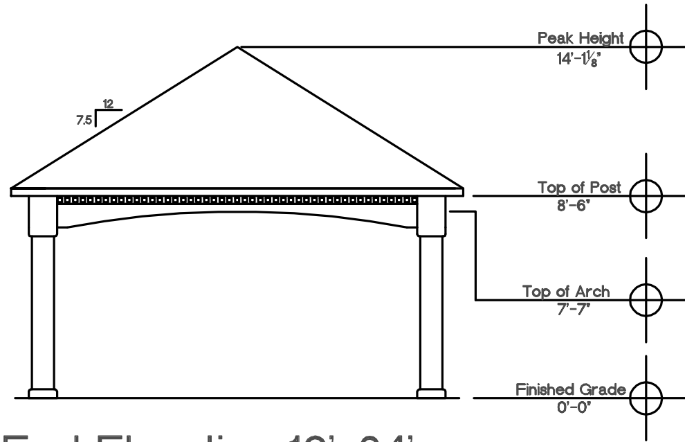
End Elevation 16'x24'
