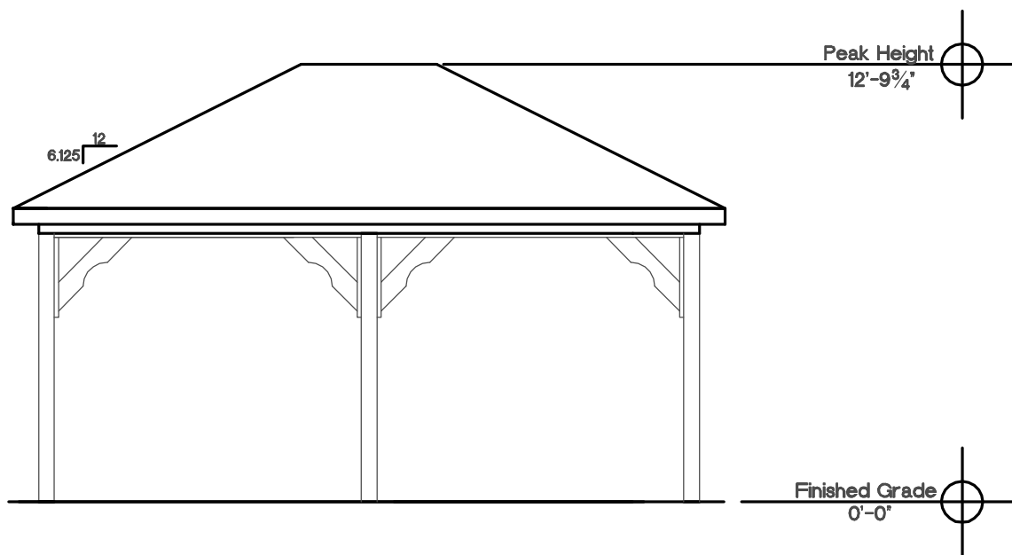
Side Elevation 16'x20' N.T.S.
