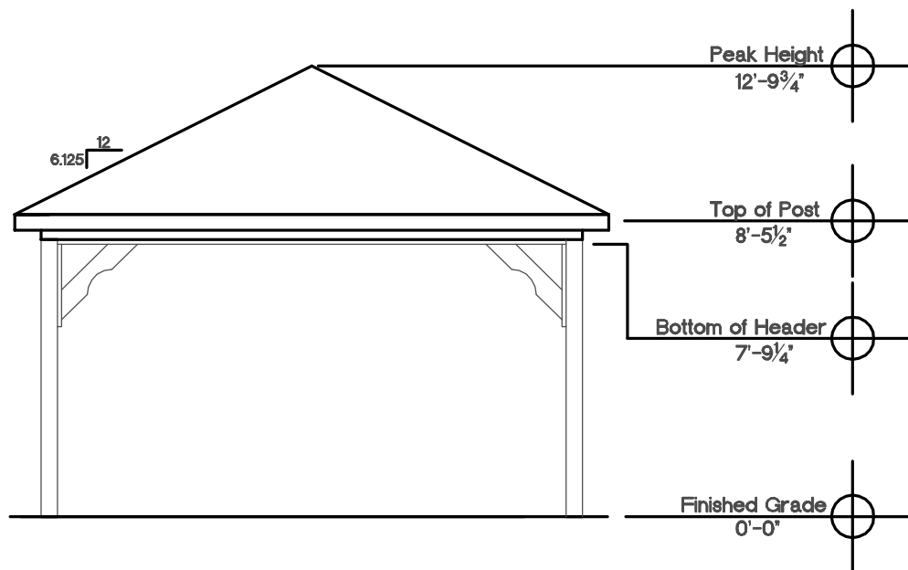
End Elevation 16'x20' N.T.S.
