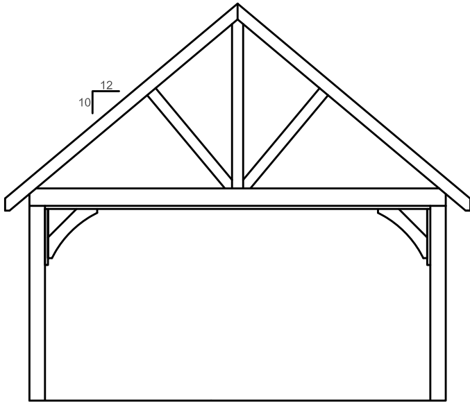
End Elevation
