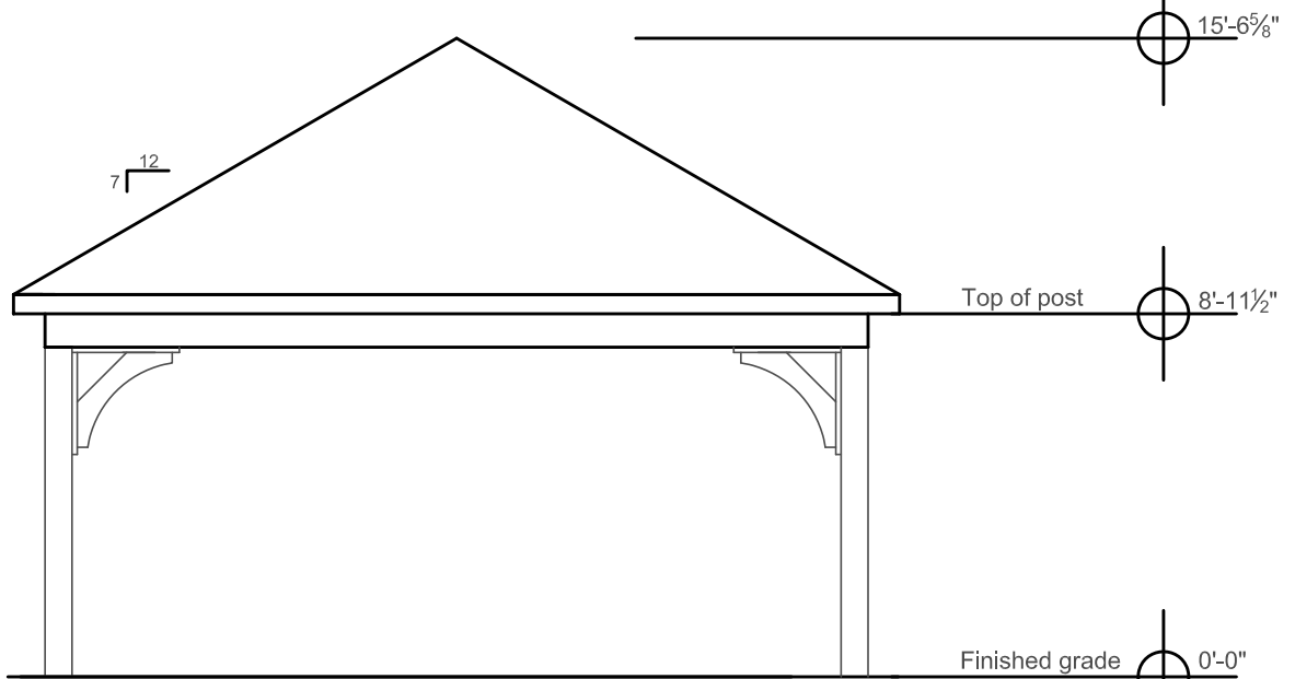
End Elevation
