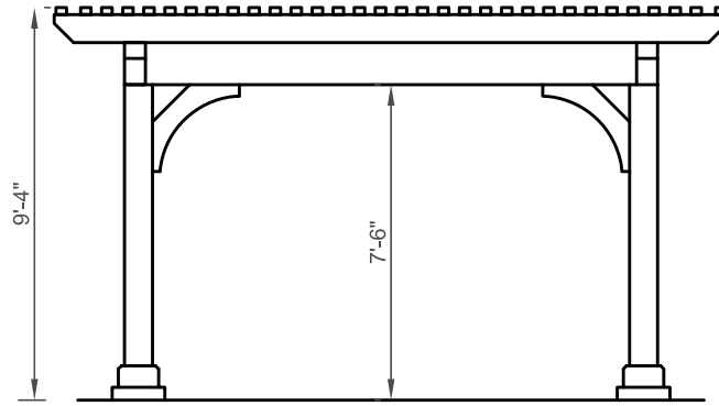
End Elevation
