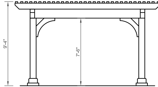
End Elevation
