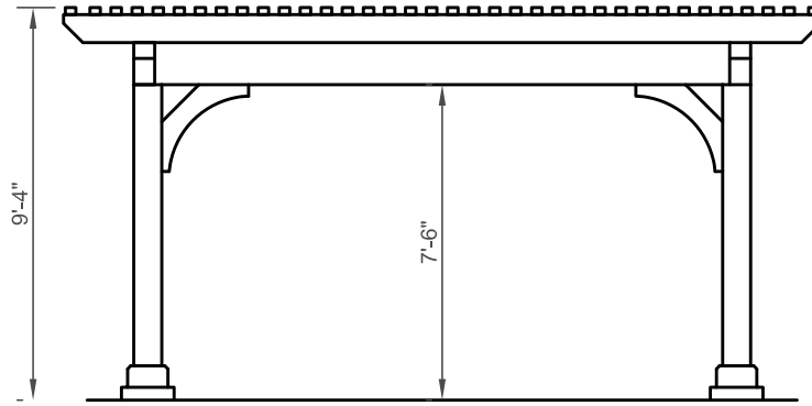
End Elevation
