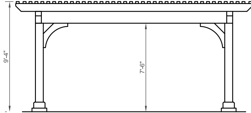
End Elevation
