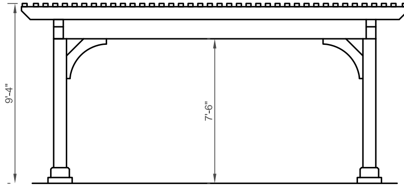
End Elevation
