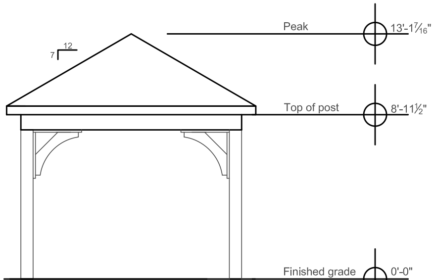
End Elevation
