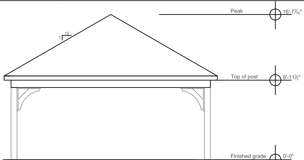
End Elevation
