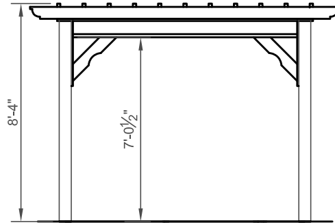
End Elevation
