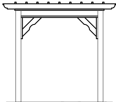
End Elevation
