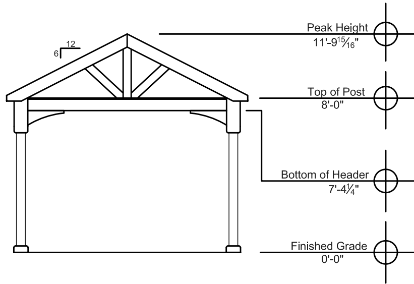
End Elevation
