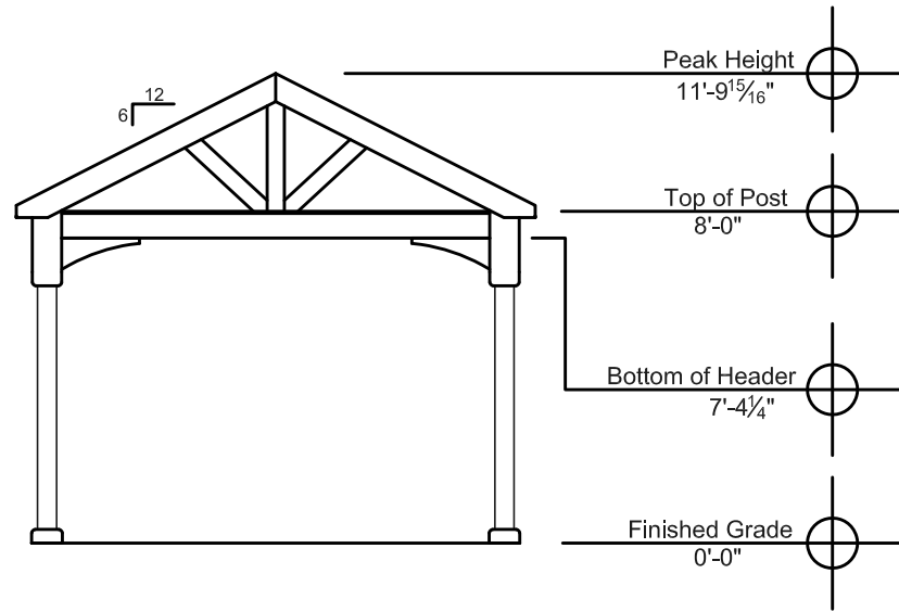
End Elevation
