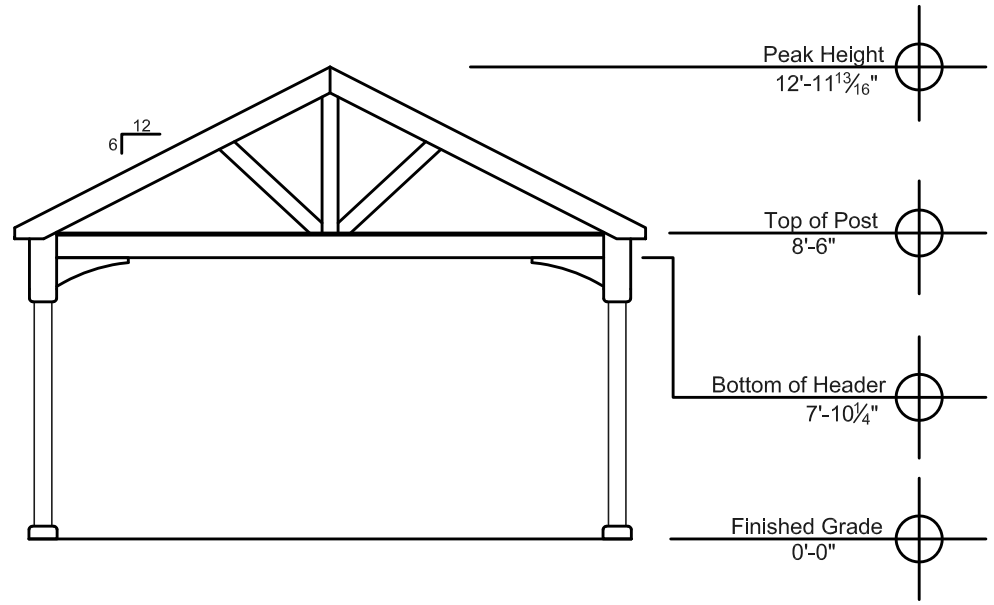
End Elevation
