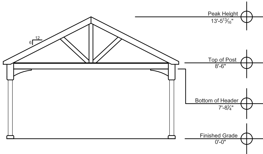
End Elevation
