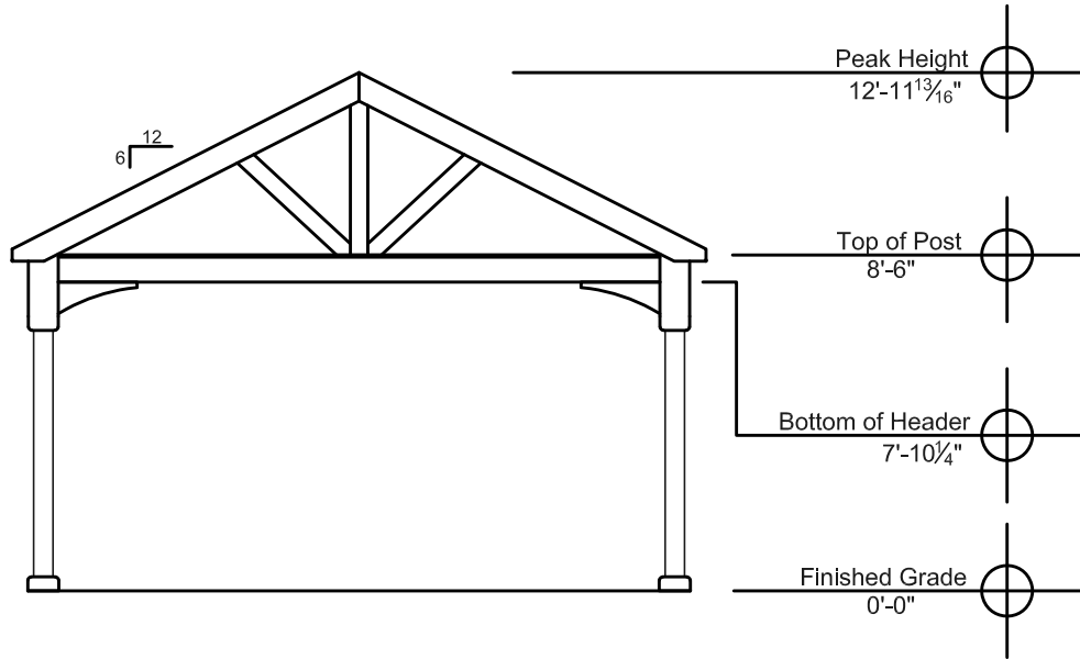
End Elevation
