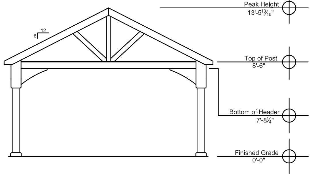
End Elevation
