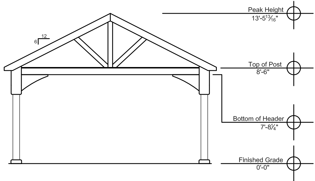
End Elevation
