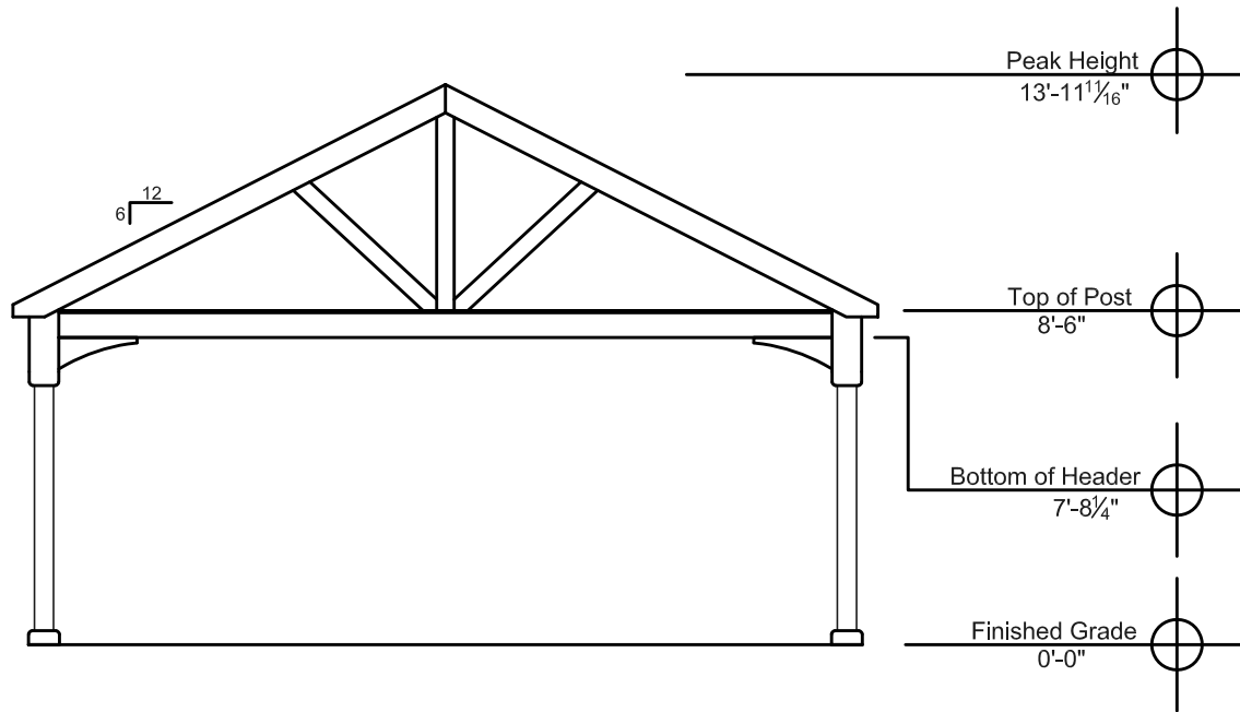
End Elevation
