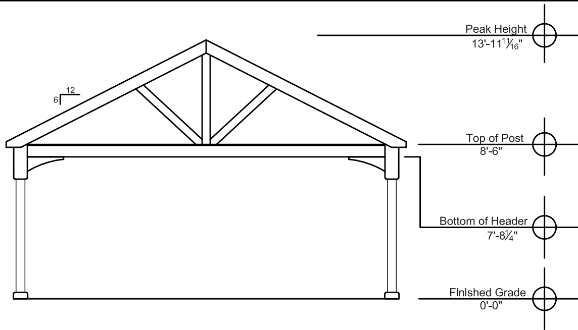
End Elevation
