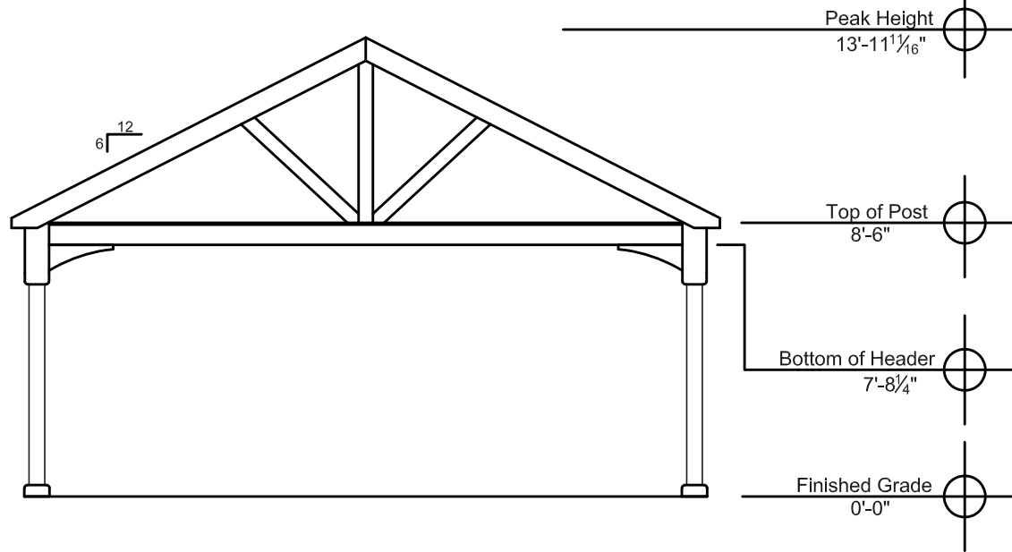
End Elevation
