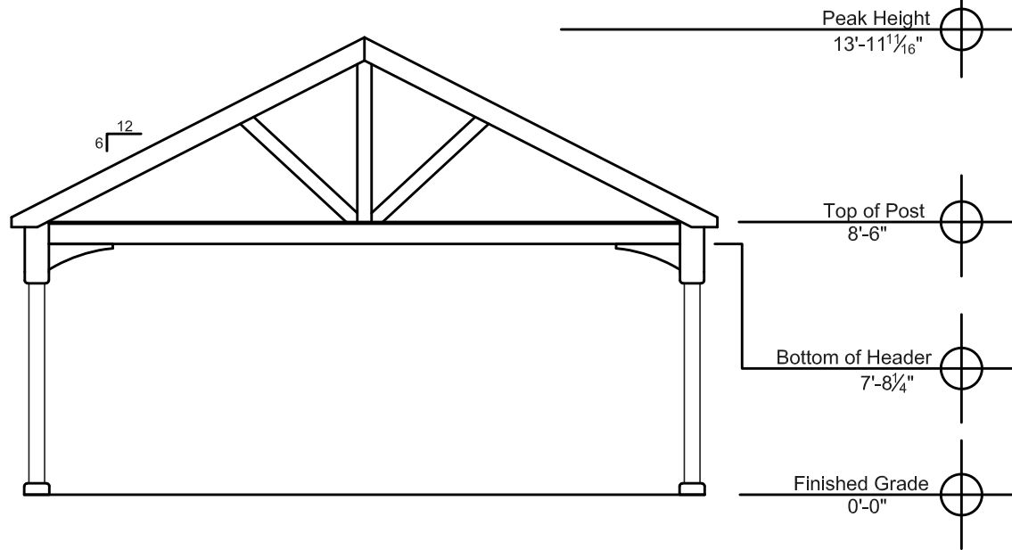
End Elevation
