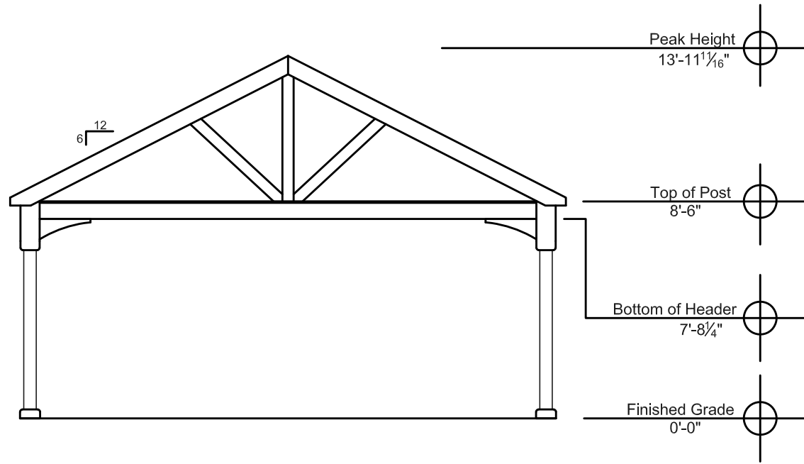
End Elevation
