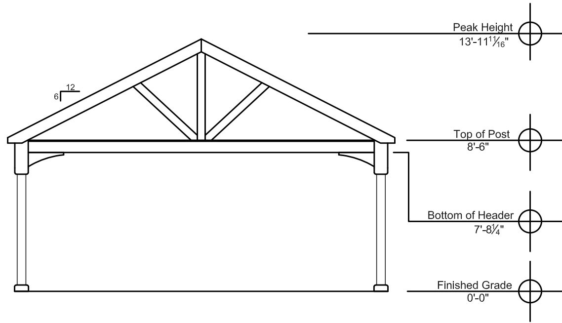
End Elevation
