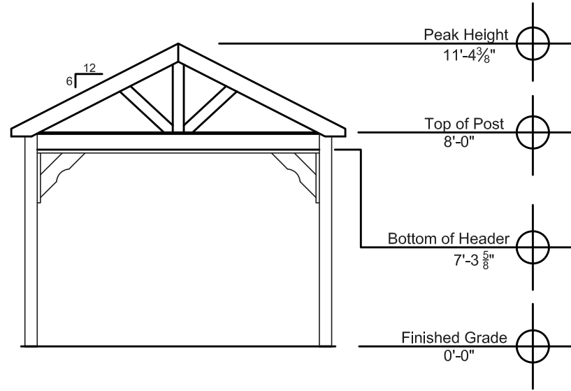
End Elevation
