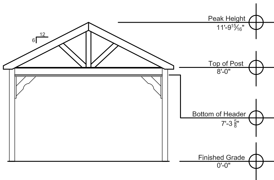
End Elevation
