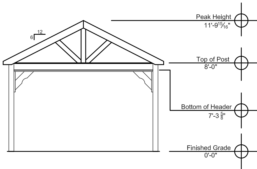
End Elevation
