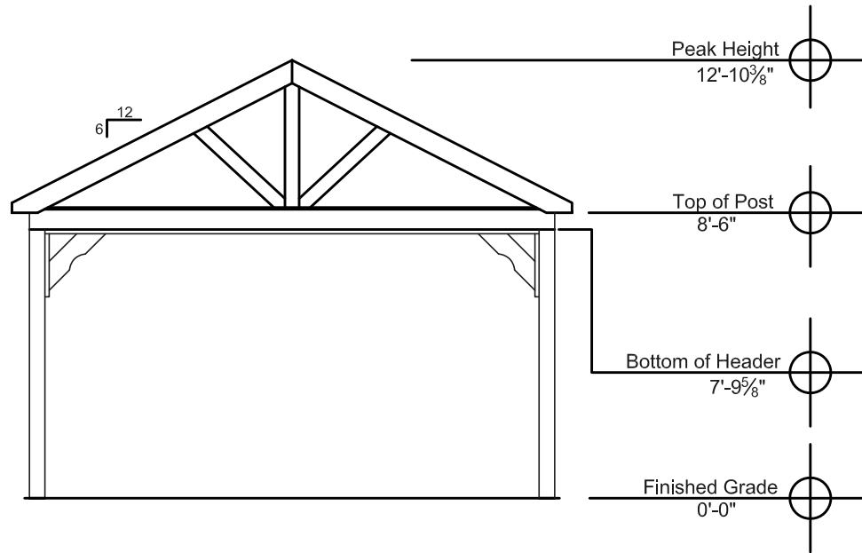
End Elevation
