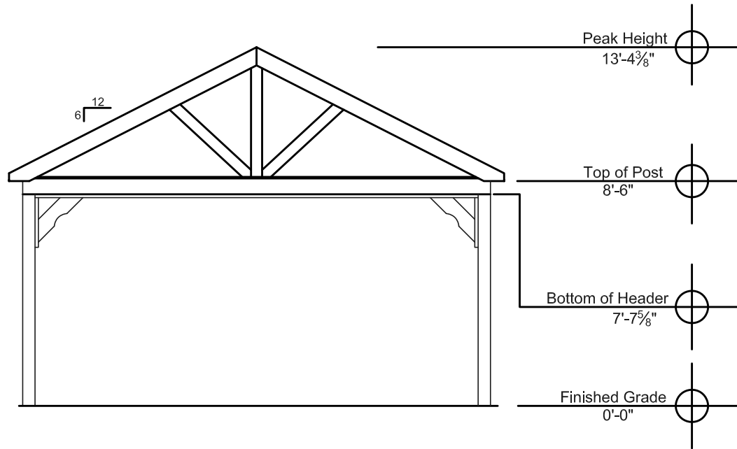
End Elevation
