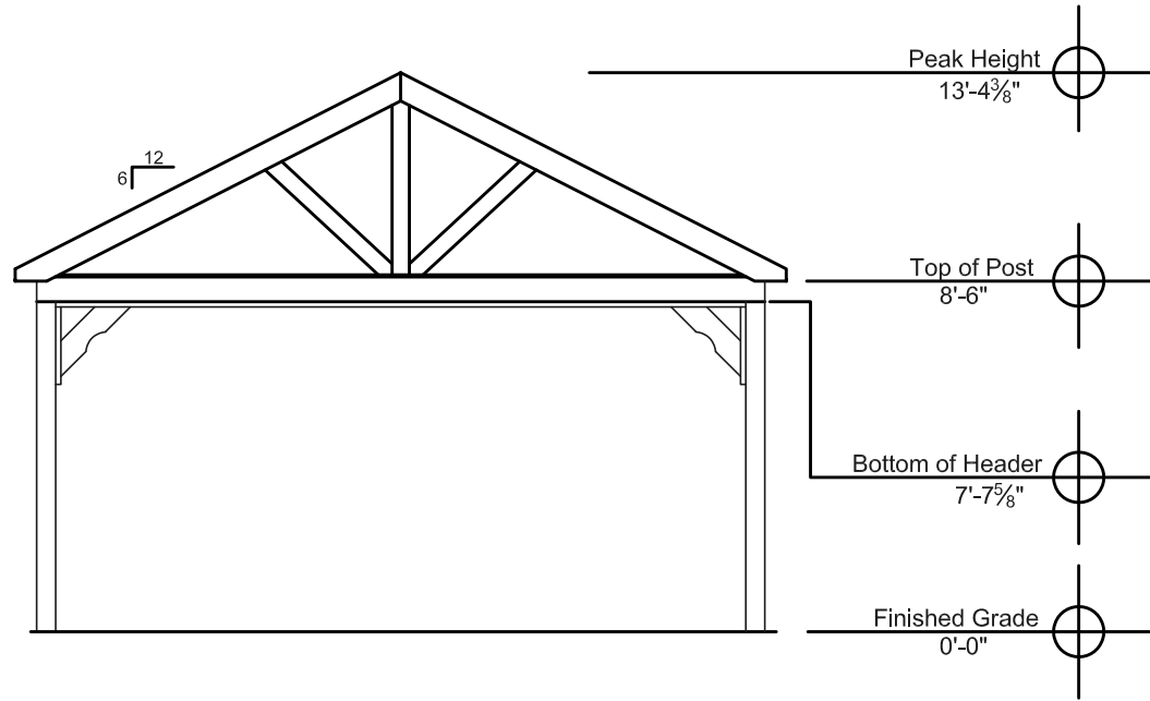
End Elevation
