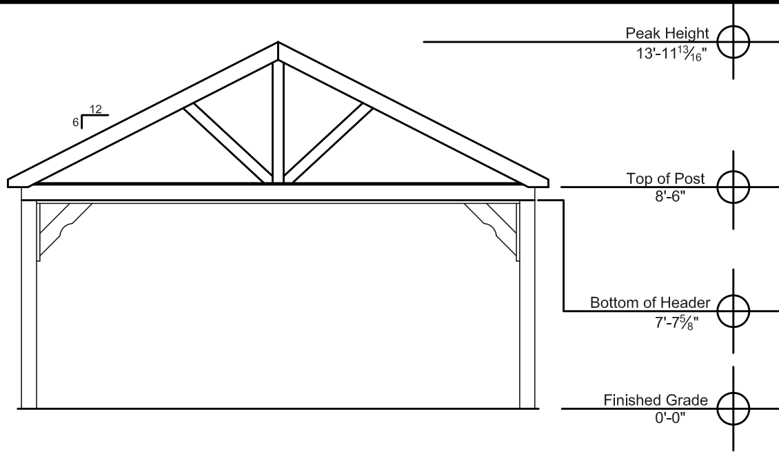
End Elevation
