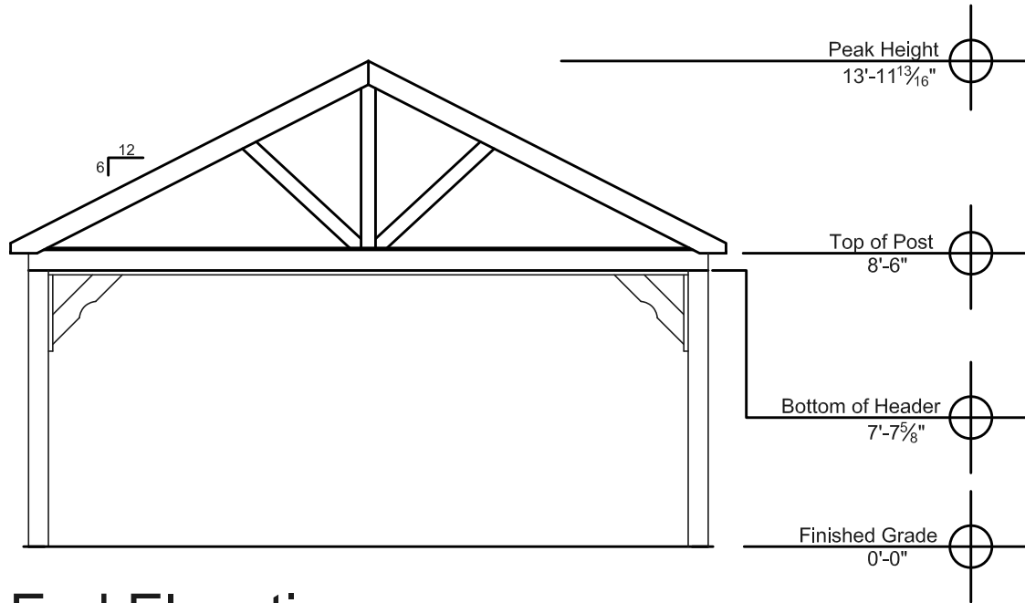
End Elevation
