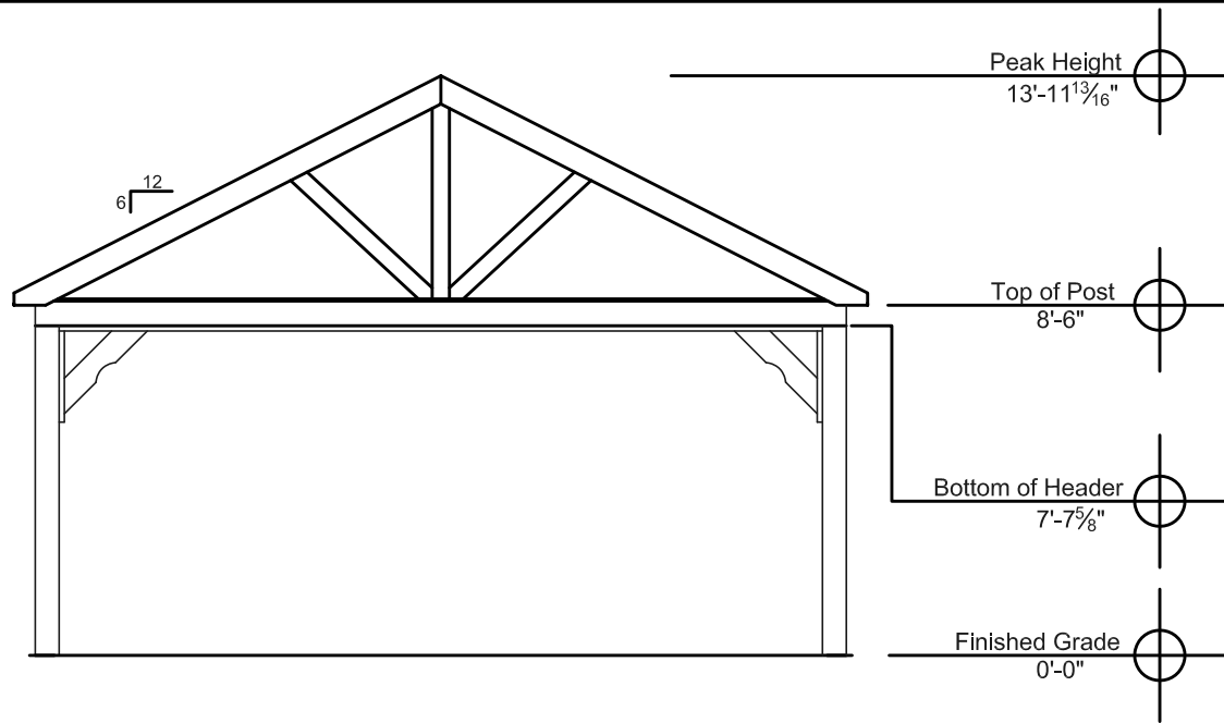
End Elevation
