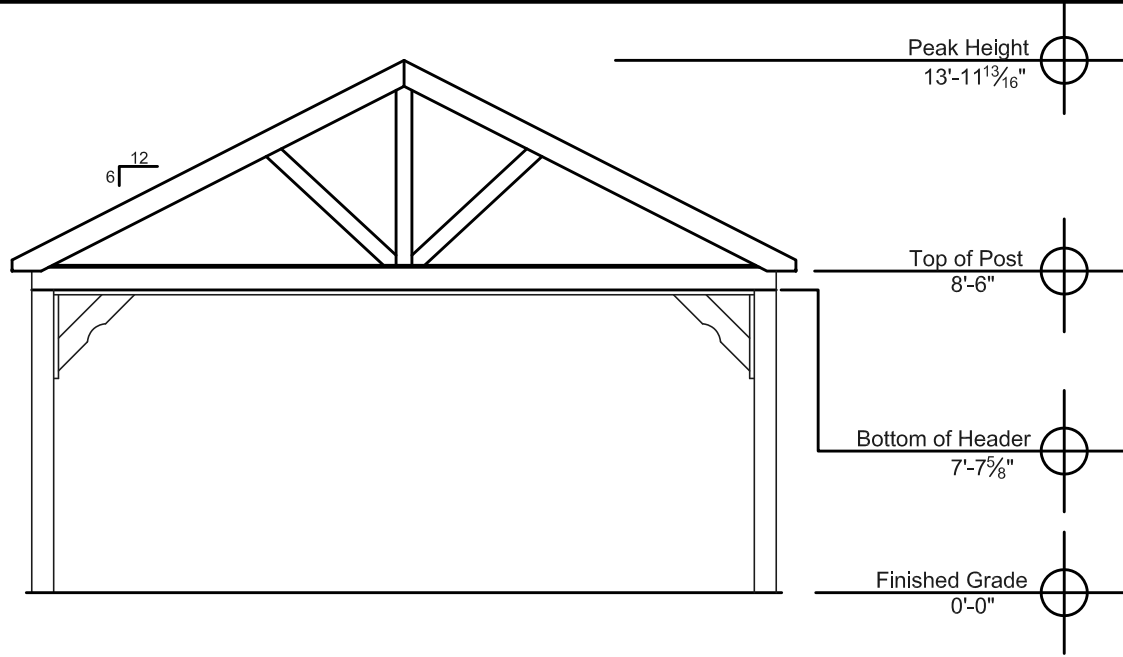
End Elevation
