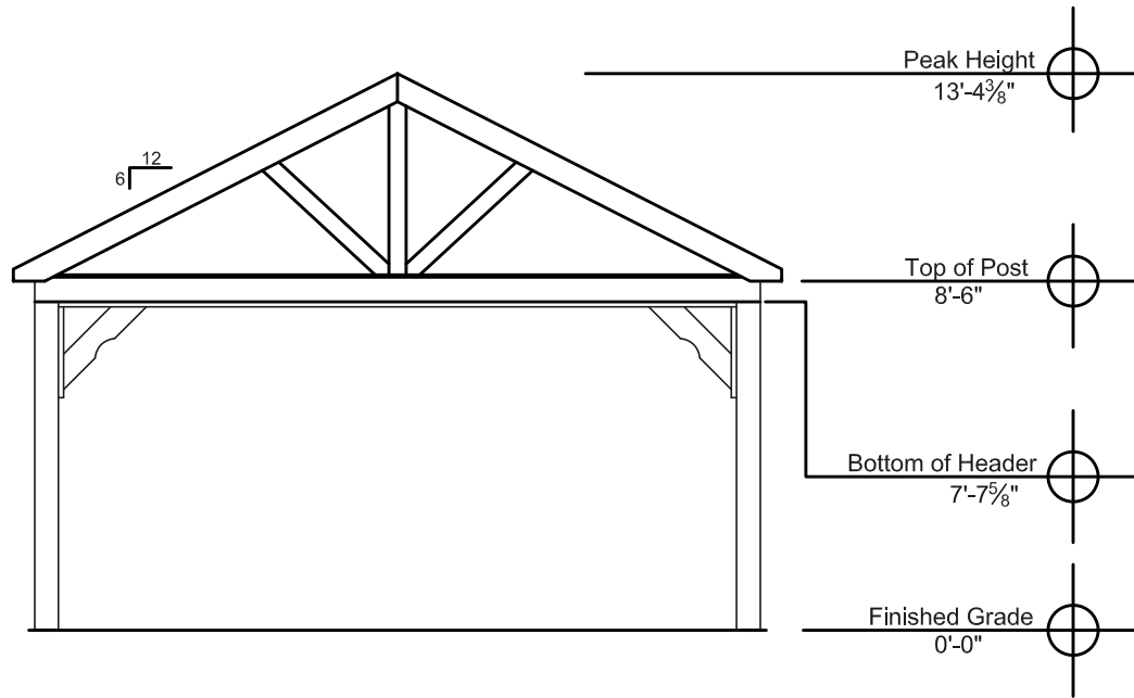
End Elevation
