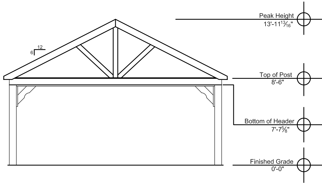
End Elevation
