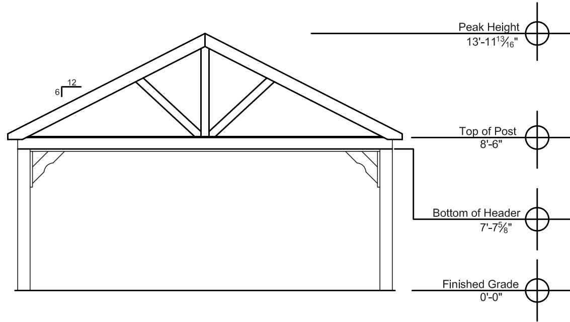
End Elevation
