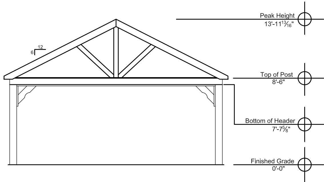
End Elevation
