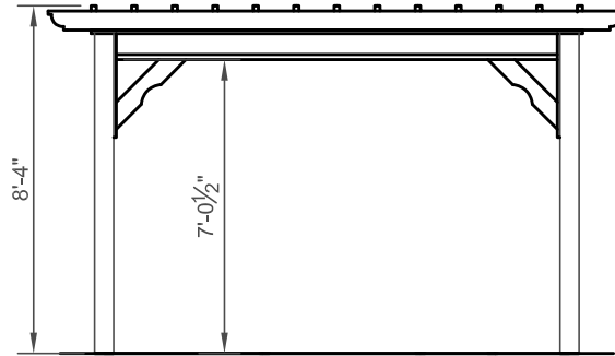
End Elevation
