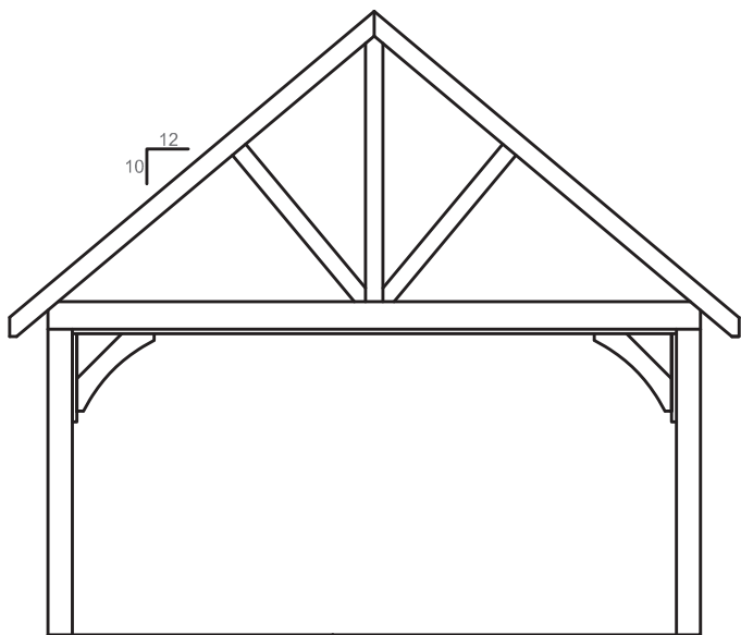
End Elevation
