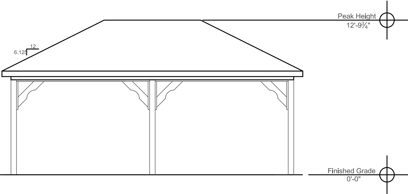
Side Elevation 16'x24' N.T.S.
