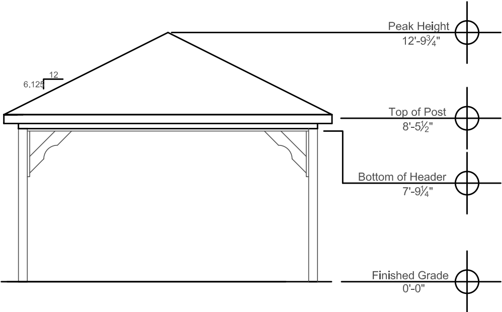
End Elevation 16'x24' N.T.S.
