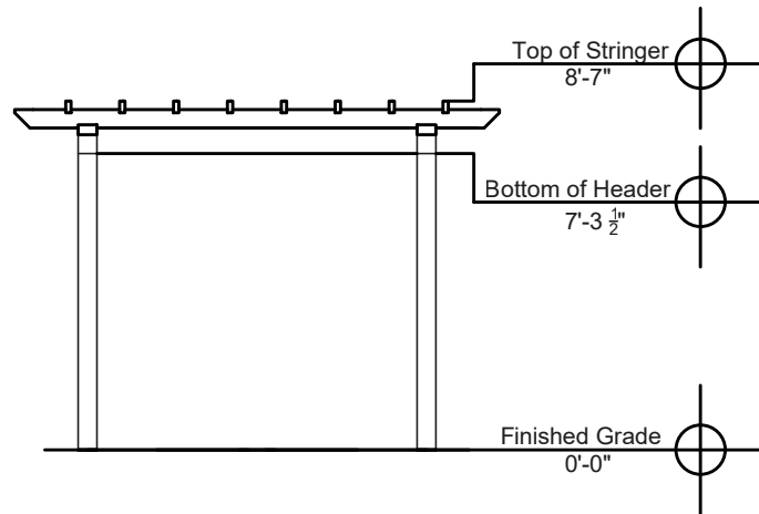
End Elevation
