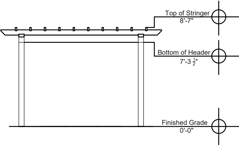
End Elevation
