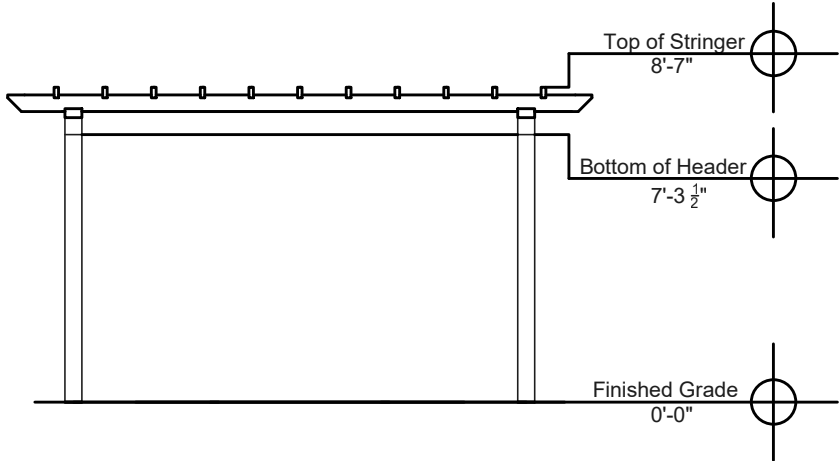
End Elevation
