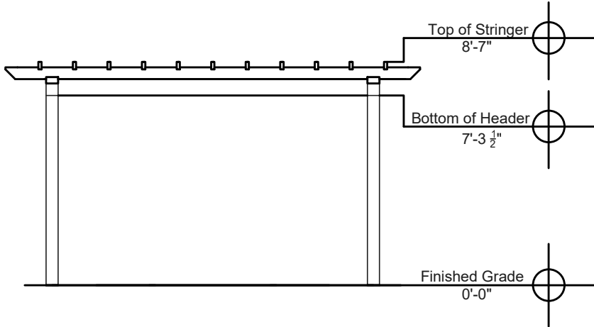
End Elevation
