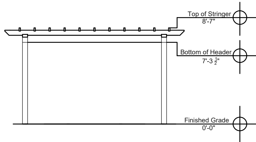
End Elevation
