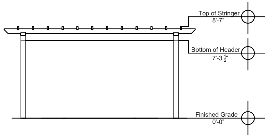
End Elevation
