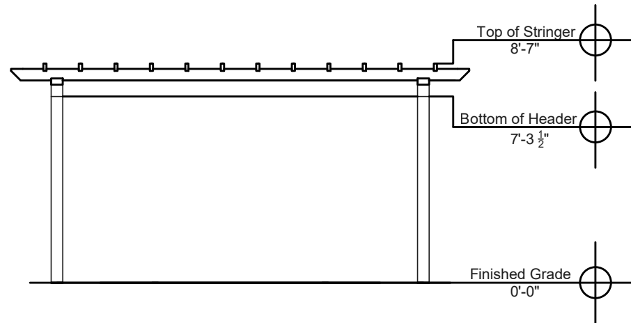
End Elevation
